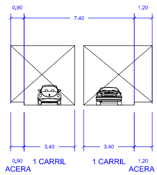
TUNEL DE ACCESO AL MUELLE DEPORTIVO.
