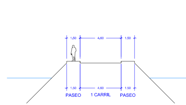
VIARIO DIQUE NORTE (MUELLE DEPORTIVO OESTE).
