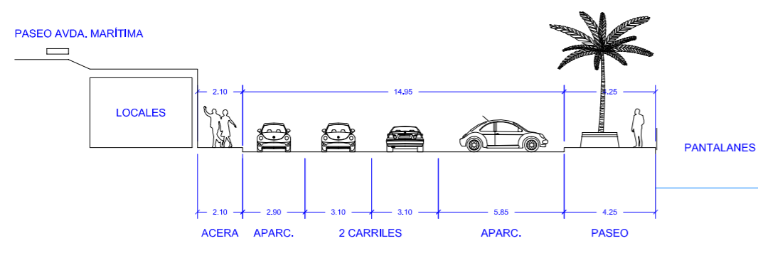
TRAMO 2 VIARIO C/ JOAQUIN BLANCO TORRENT (MUELLE DEPORTIVO OESTE).
