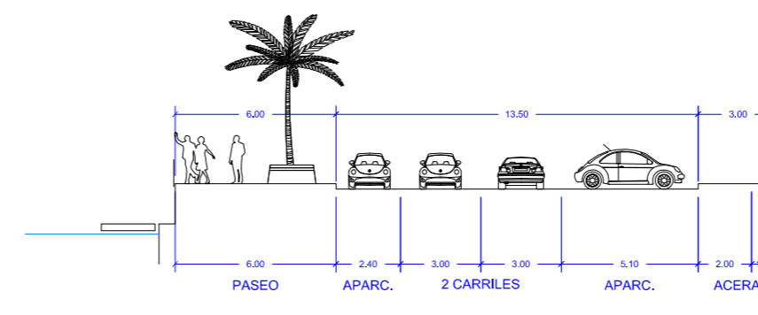
VIARIO DE DIQUE ESTE (MUELLE DEPORTIVO ESTE).
