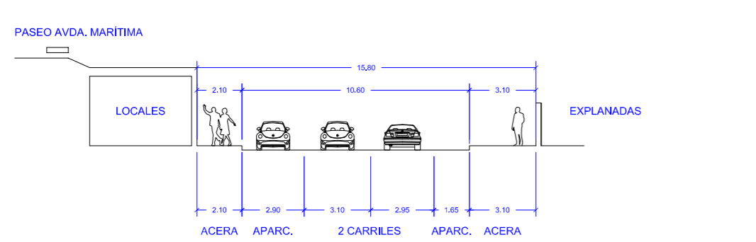
TRAMO 2 VIARIO C/ JOAQUIN BLANCO TORRENT (MUELLE DEPORTIVO OESTE).
