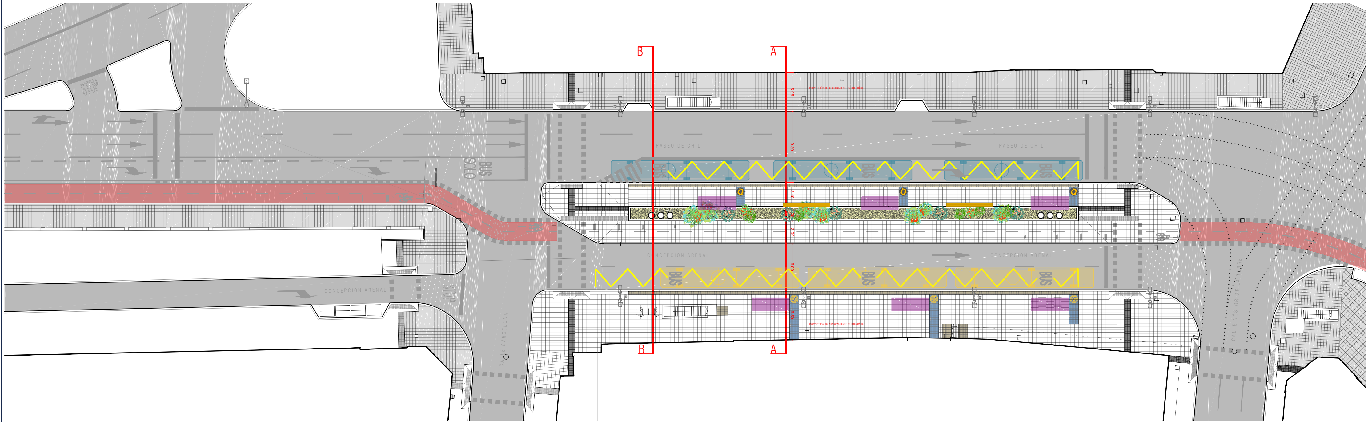
Planta General / Estado Propuesta
