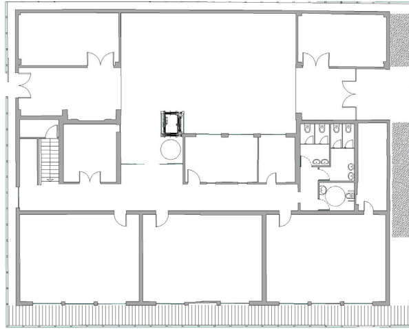
PLANTA 0
